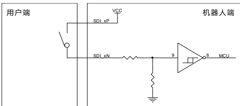
图 6-20 电气原理图
