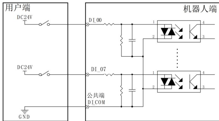
图 6-15 电气原理图
