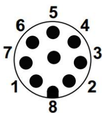
图 6-28 末端圆形连接器接口定义
