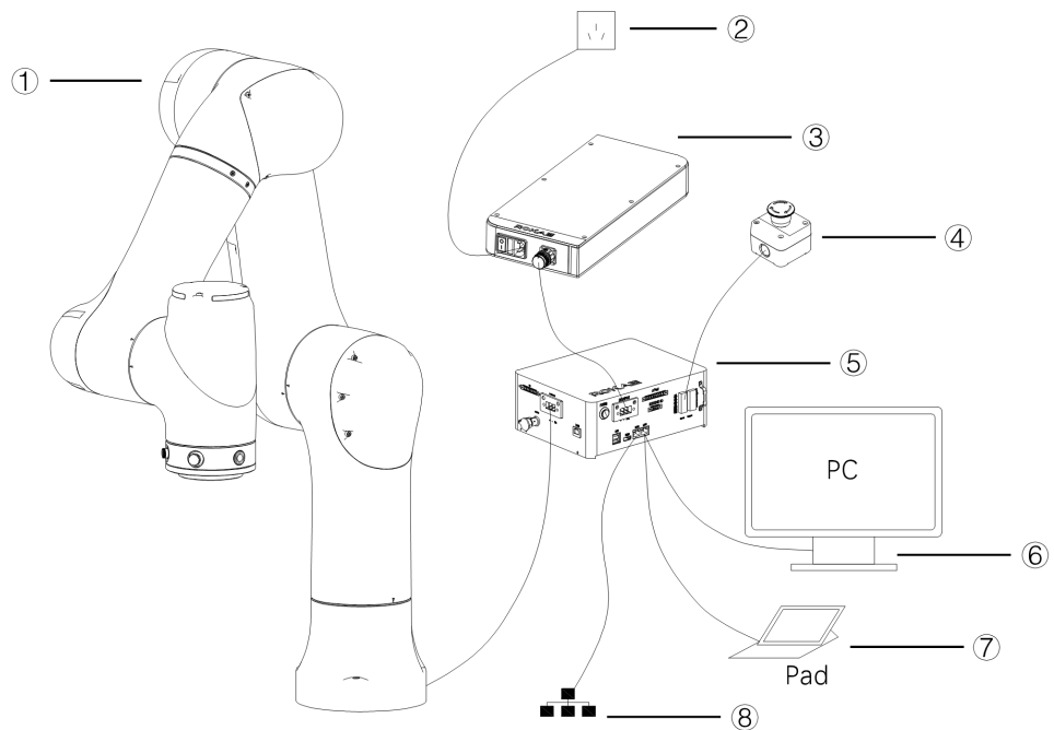
图 6-1 电气布局图
