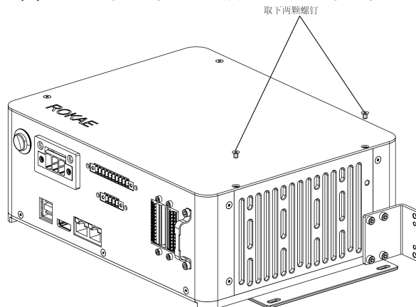
图 5-10 拆卸螺钉
