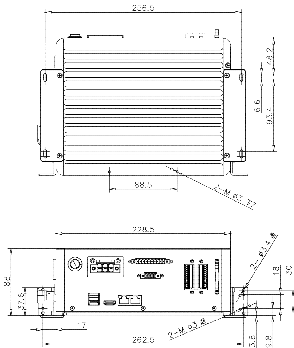
图 5-7 卧式安装
