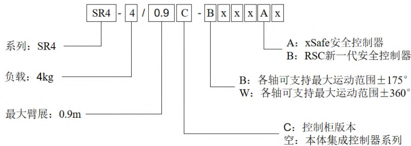
图 4-1 SR4-4/0.9C 机型型号说明
