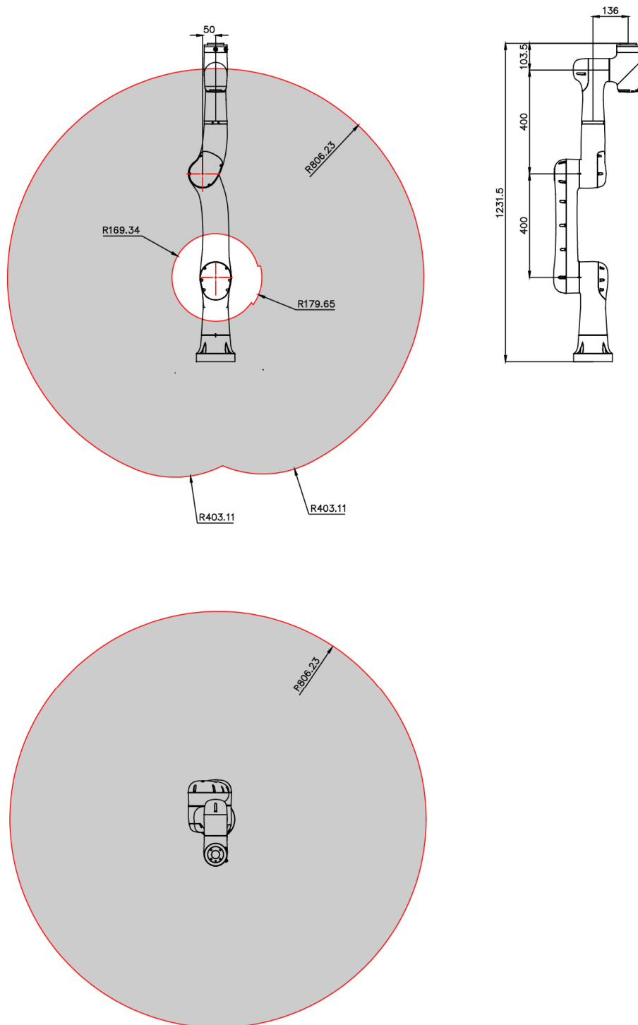
图 4-2 SR4-4/0.9C 工作空间图
