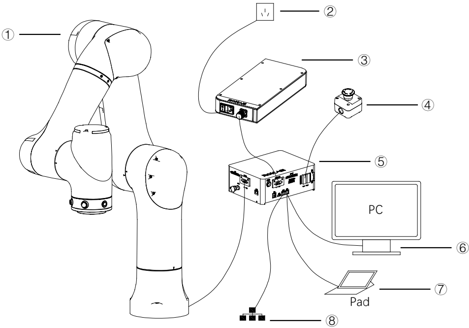
图 6-1 电气布局图
