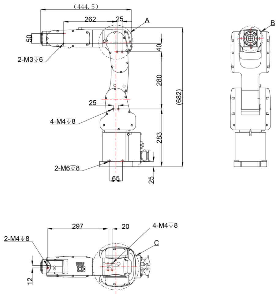
图 12 NB4-4/0.58 外形尺寸及机械接口图
