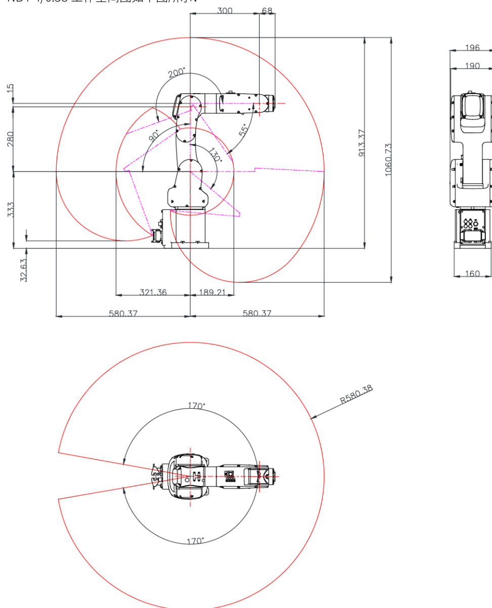
图 9 NB4-4/0.58 工作空间图
