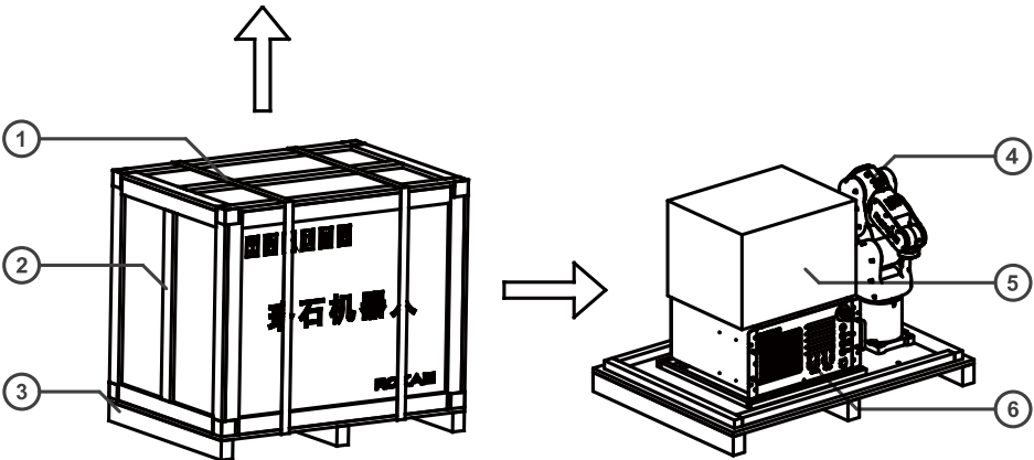
图 16 木箱拆箱示意图
