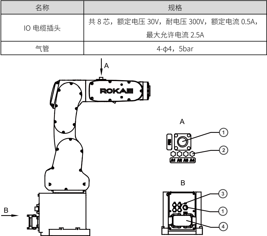
图 29 用户配线配管图
