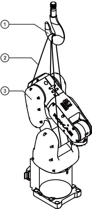
图 21 机器人吊装搬运
