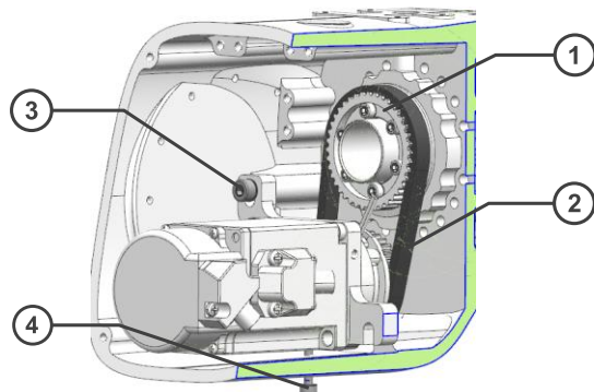
图 39 同步带维护
