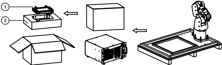
图 17 控制柜及示教器纸箱拆箱图
