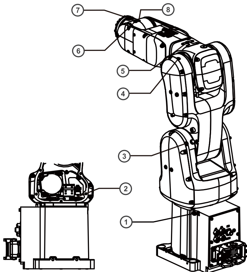
图 34 注油位置示意图
