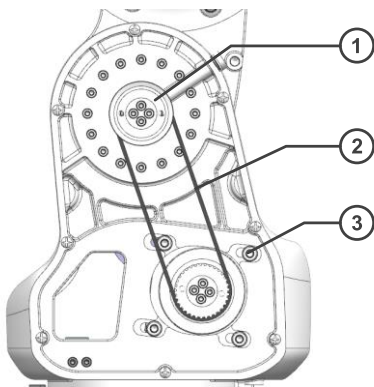
图 37 同步带维护
