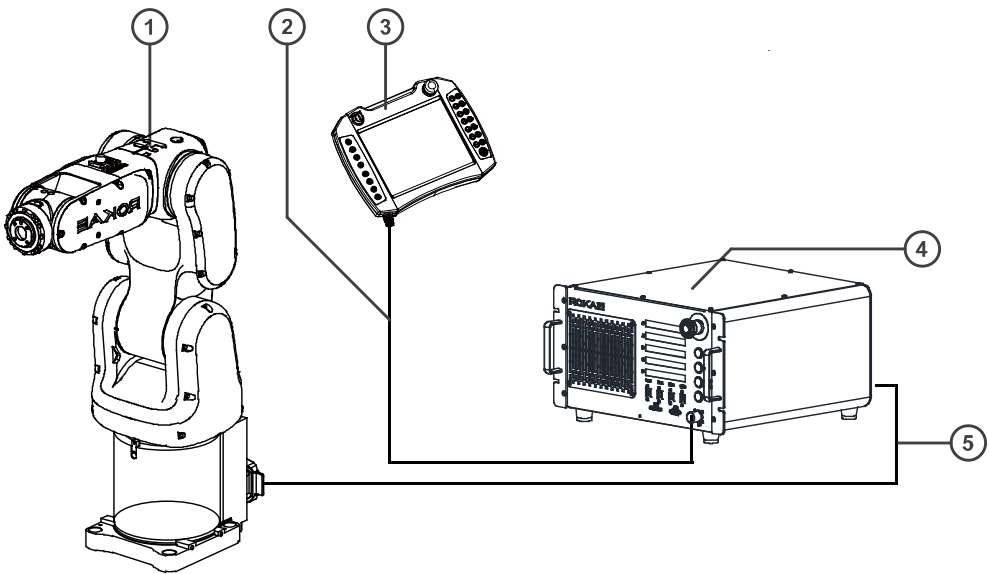
图 2 机器人系统
