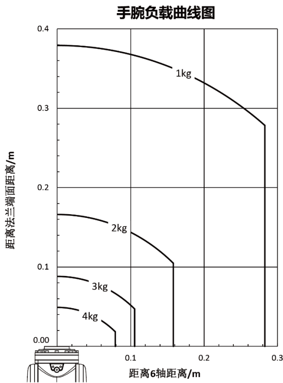
图 7 NB4-4/0.47、NB4-4/0.58、NB4h-4/0.58 手腕负载图
