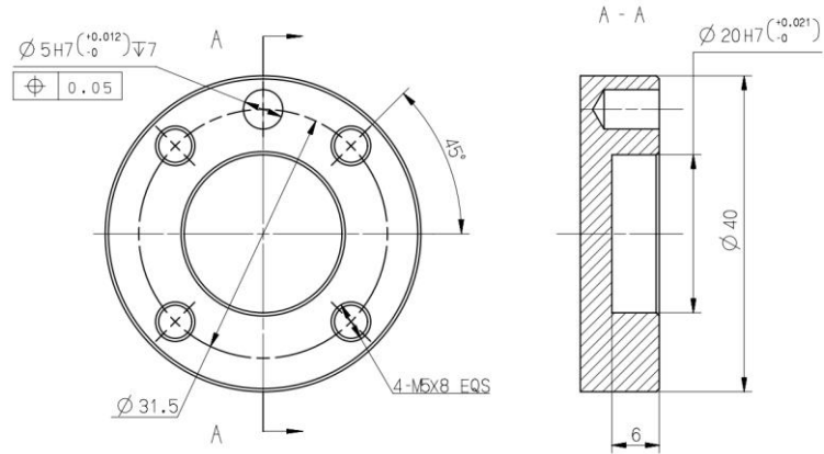
图 14 标准手腕输出法兰图
