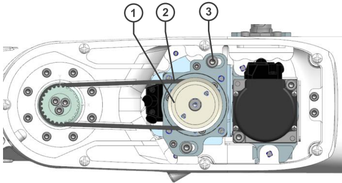
图 40 同步带维护
