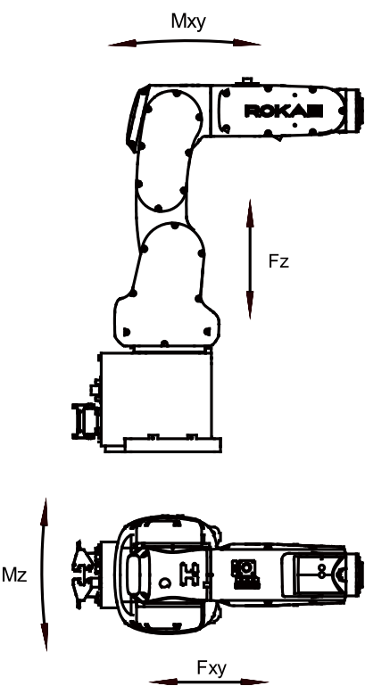
图 25 机器人支反力图
