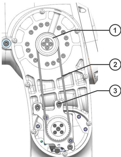
图 38 同步带维护
