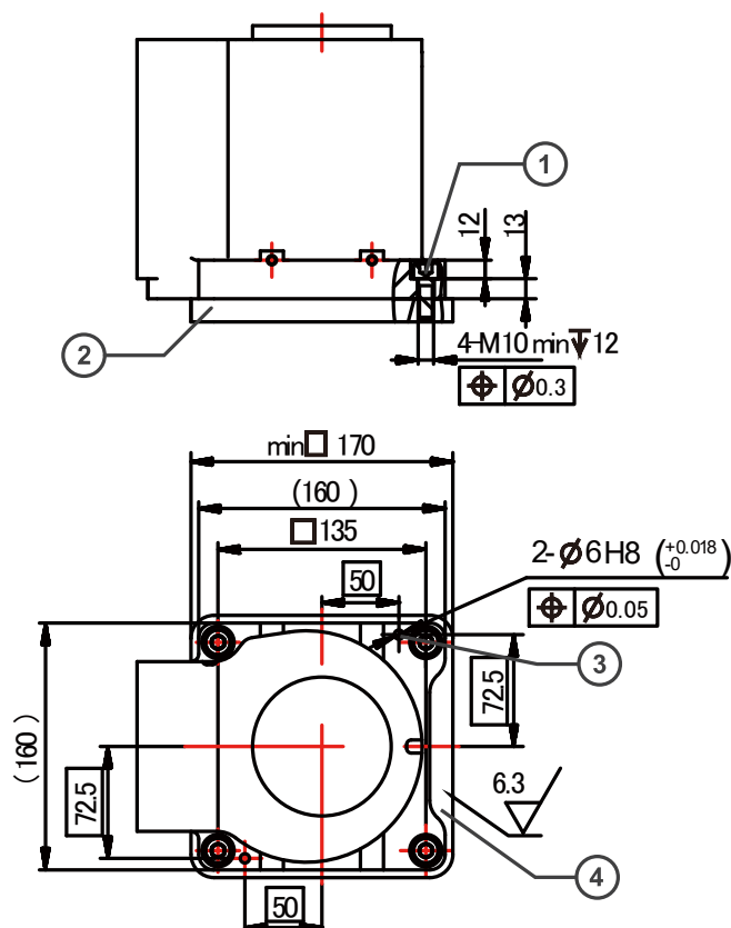
图 23 支架固定方式
