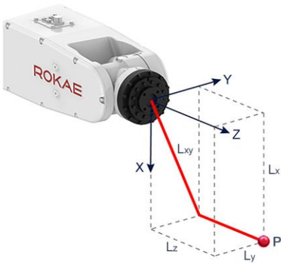
图 6 负载重心
