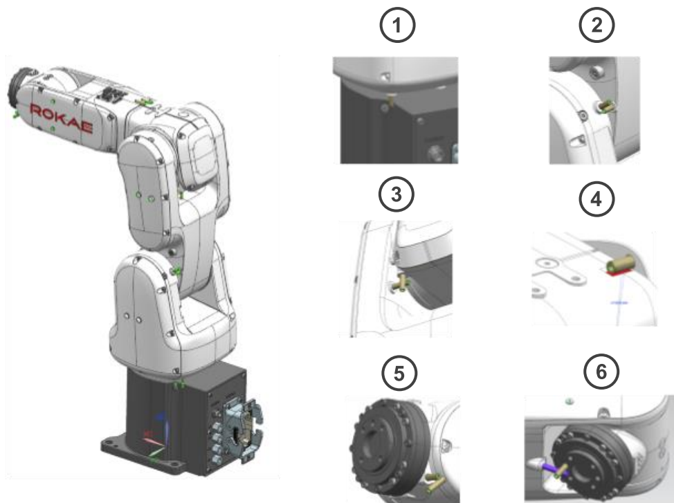
图 30 标定方法
