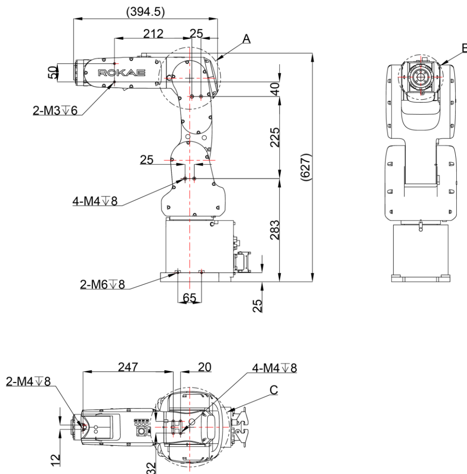
图 11 NB4-4/0.47 外形尺寸及机械接口图
