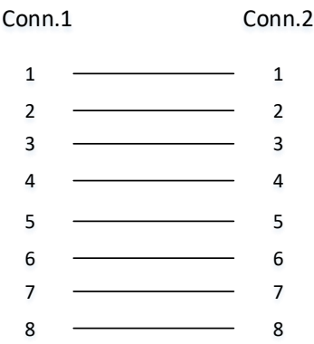
图 28 机器人内部 IO 连接电气图
