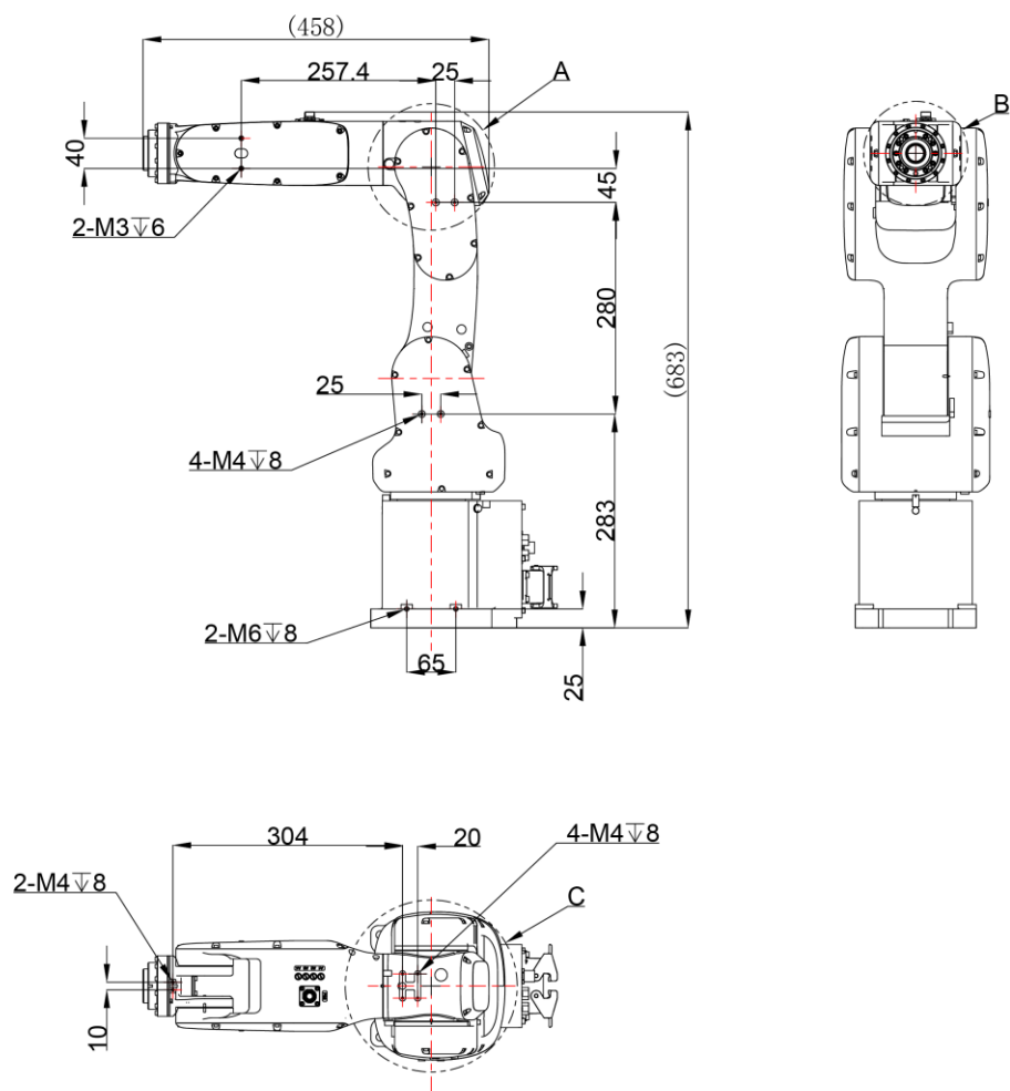
图 13 NB4h-4/0.58 外形尺寸及机械接口图
