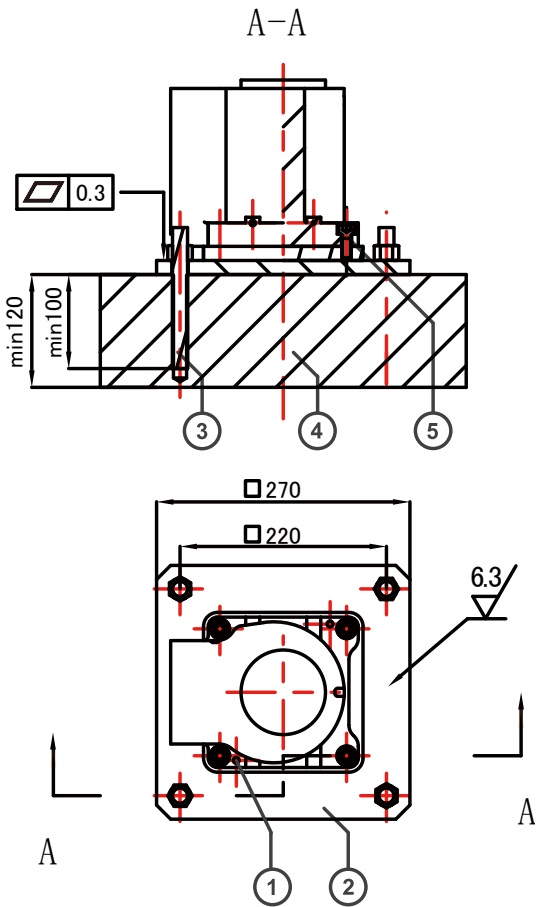
图 24 地基固定方式
