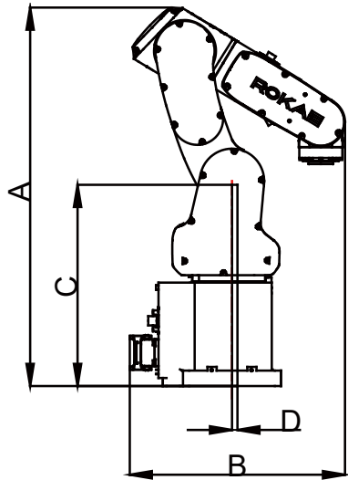
图 20 NB4 系列机器人搬运参考尺寸
