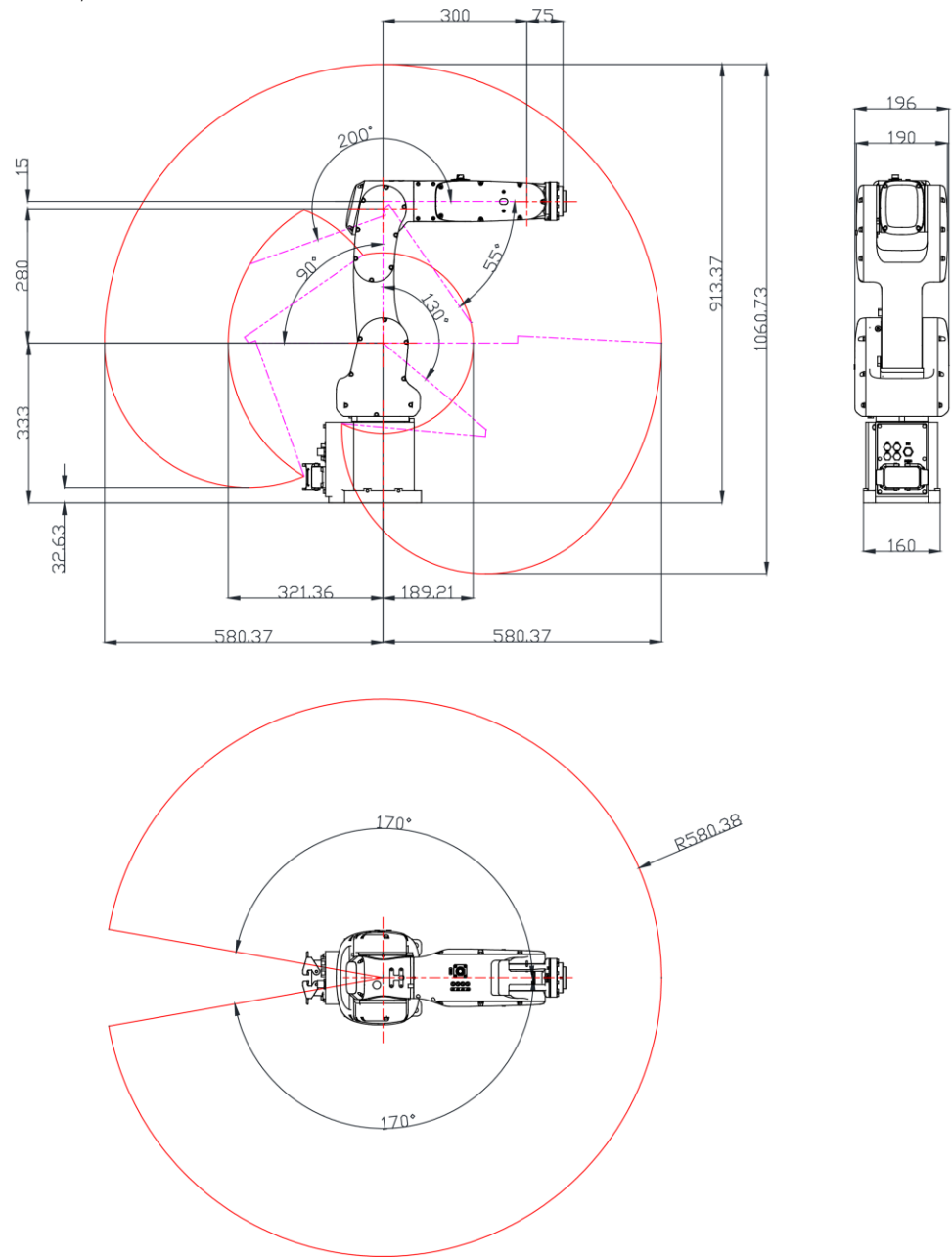
图 10 NB4h-4/0.58 工作空间图
