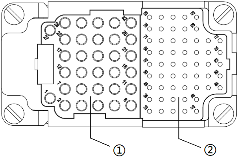
图 26 机器人本体侧端口定义图
