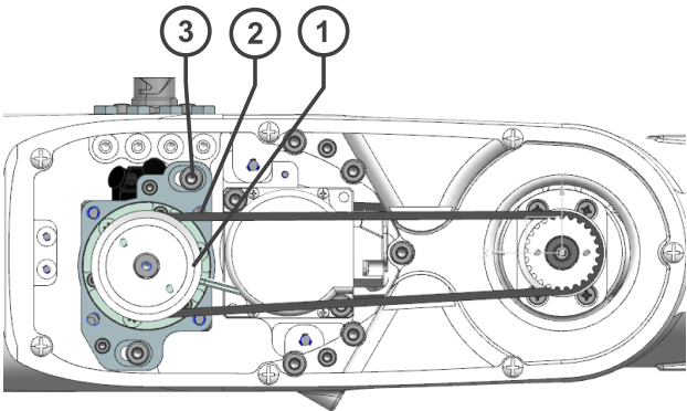
图 41 同步带维护
