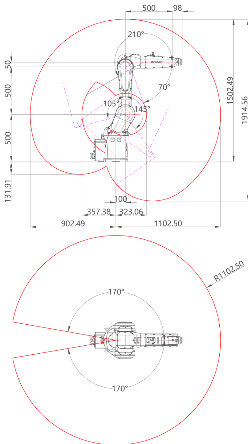
图 10 NB12-16/1.1 工作空间图
