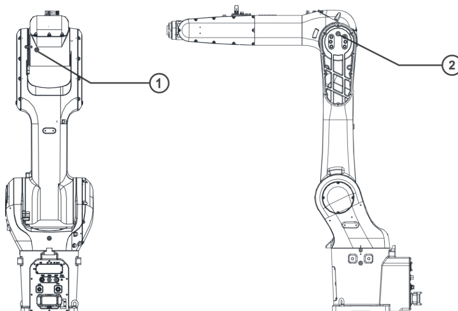
图 46 三轴减速器润滑脂加注
