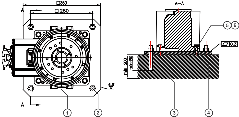
图 28 地基固定方式
