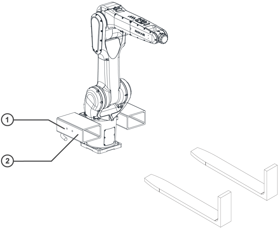
图 26 叉车搬运
