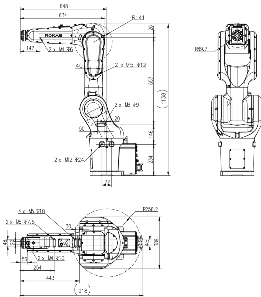
图 16 NB12-16/1.0 外形尺寸及机械接口图
