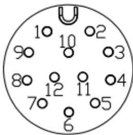
图 36 PS1 引脚定义图
