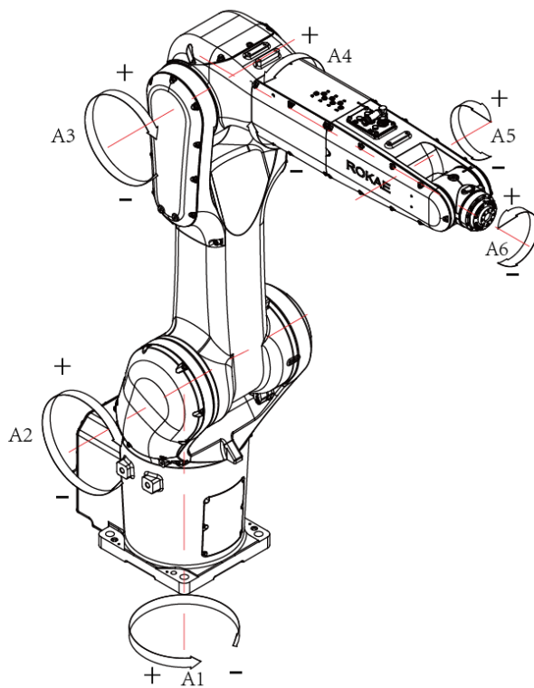
图 3 六轴机器人各轴运动方向
