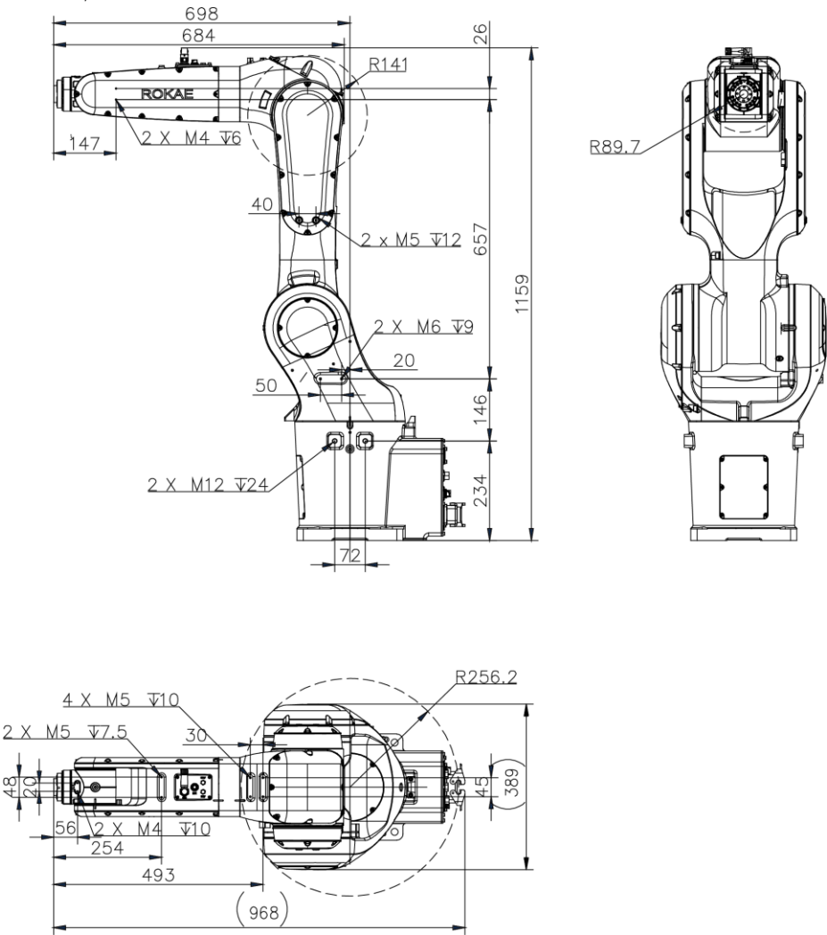
图 15 NB12-16/1.1 外形尺寸及机械接口图
