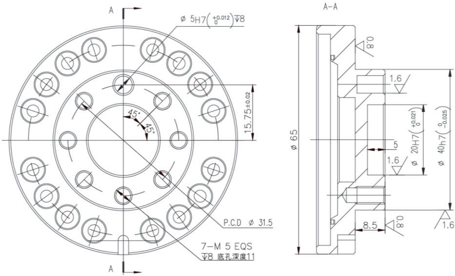
图 19 手腕输出法兰图
