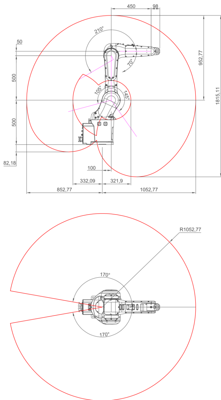
图 11 NB12-16/1.0 工作空间图
