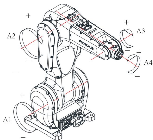
图 4 三轴和四轴机器人各轴运动方向
