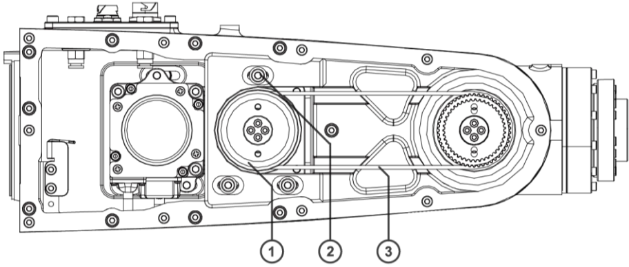
图 51 同步带维护
