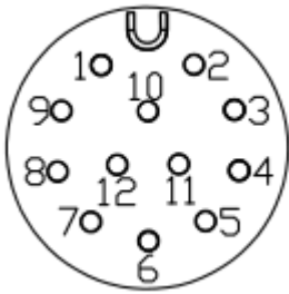
图 32 PS1、PS2 引脚定义图
