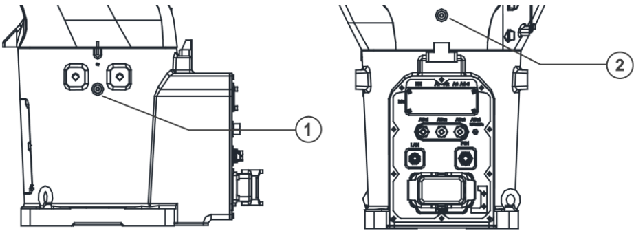
图 44 一轴减速器润滑脂加注
