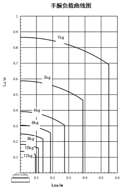
图 8 NB12 手腕负载图
