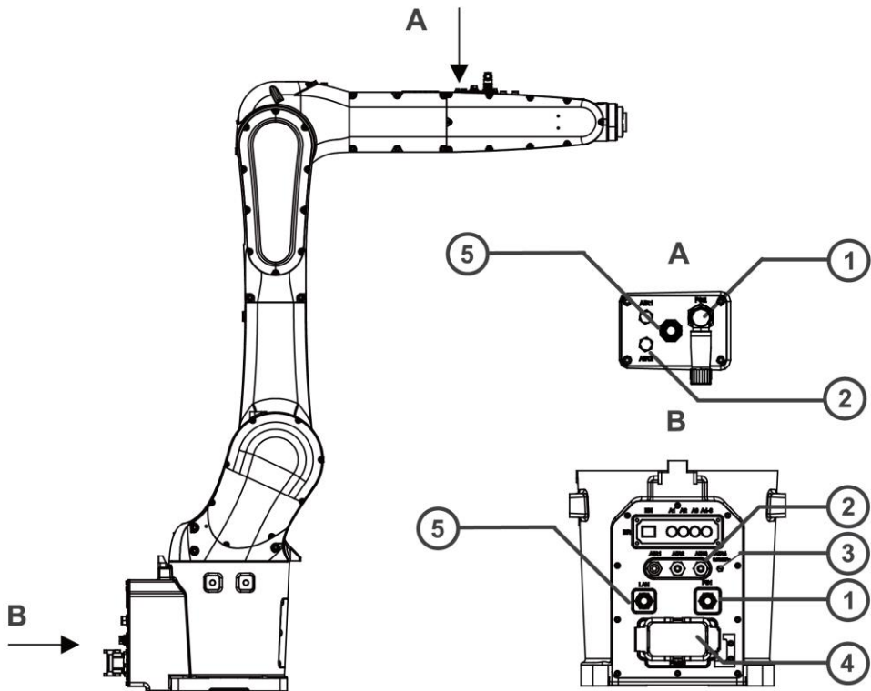
图 37 NB12-12/1.4、NB12-16/1.1、NB12-16/1.0 和 NB12-10/1.6 用户配线配管图
