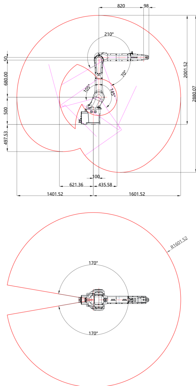
图 12 NB12-10/1.6 工作空间图
