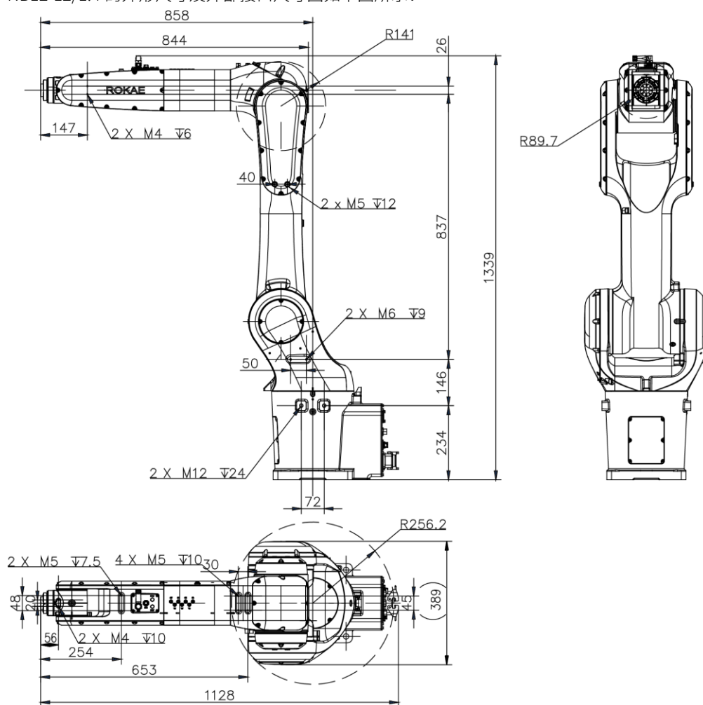
图 14 NB12-12/1.4 外形尺寸及机械接口图
