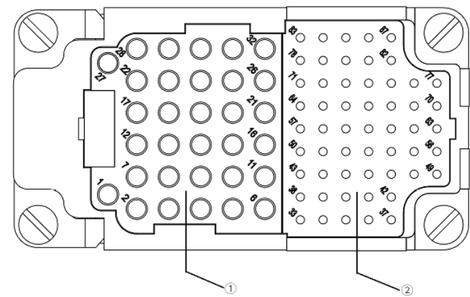
图 30 机器人本体侧端口定义图
