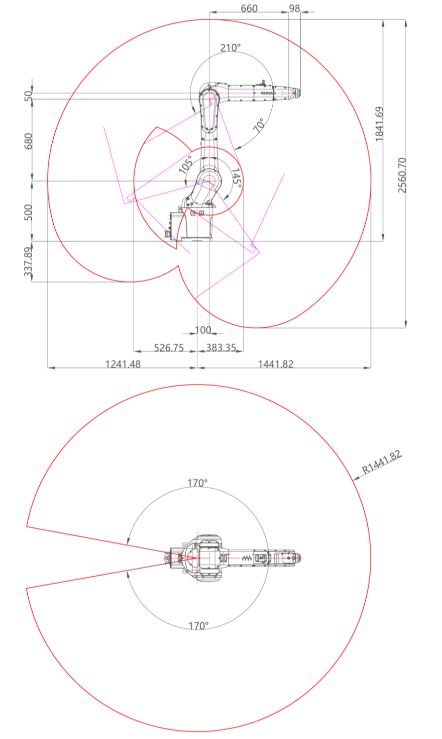
图 9 NB12-12/1.4 工作空间图
