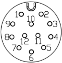
图 34 LAN 口引脚定义
