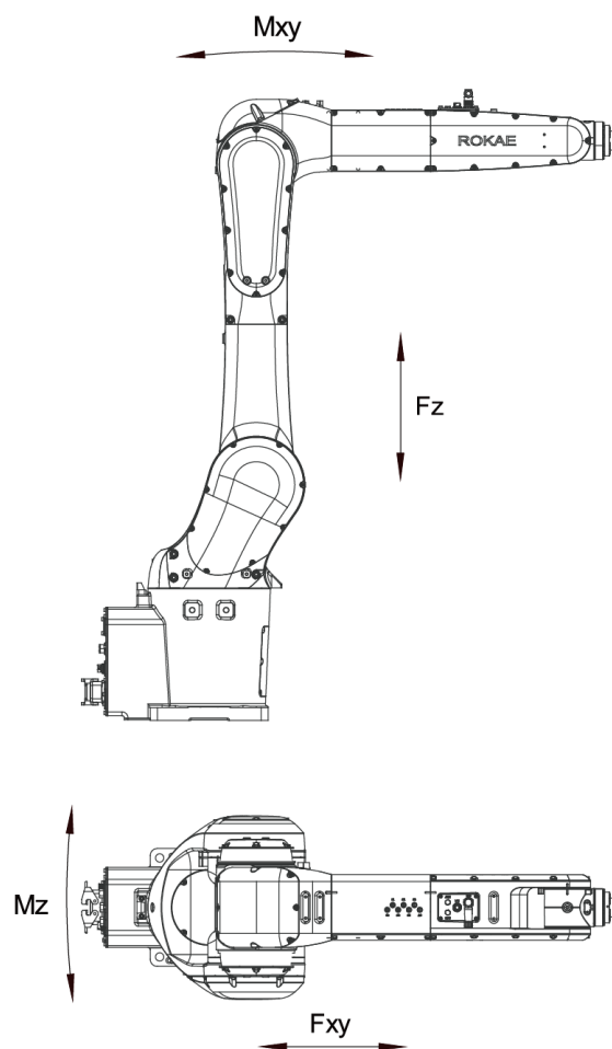
图 29 机器人支反力图
