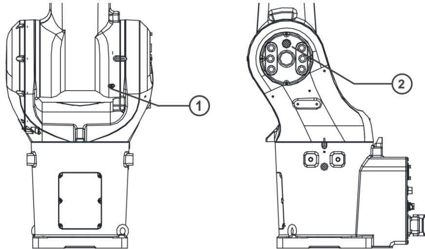
图 45 二轴减速器润滑脂加注
