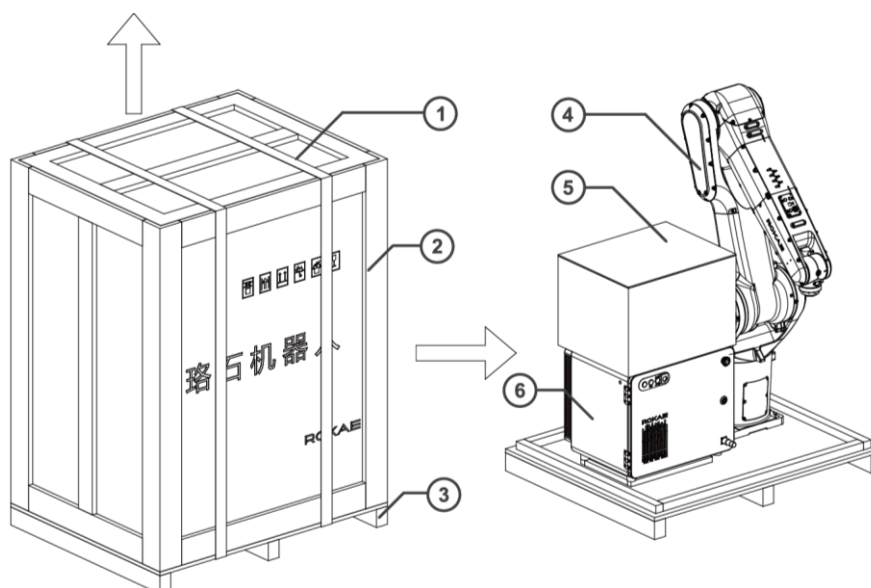
图 20 木箱拆箱示意图
