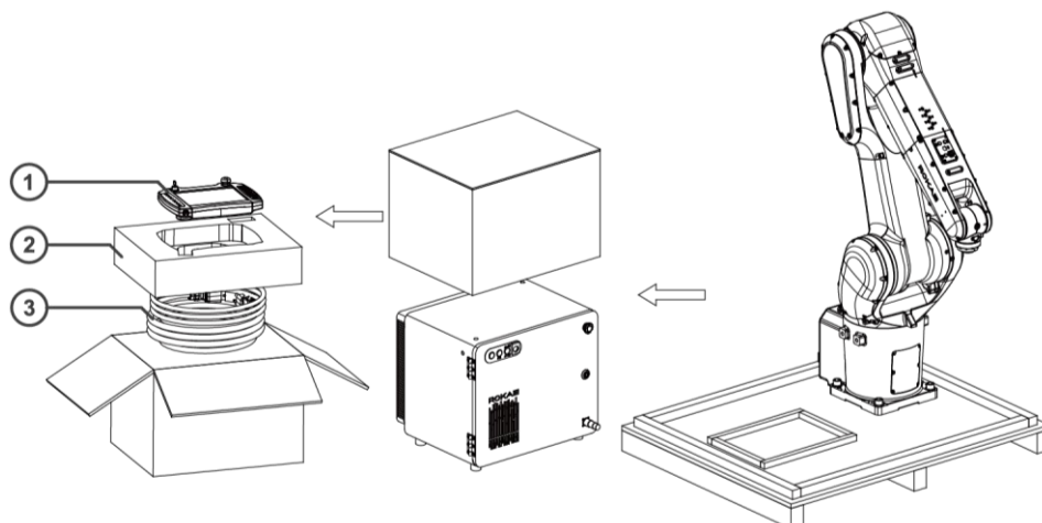
图 21 控制柜及示教器纸箱拆箱图
