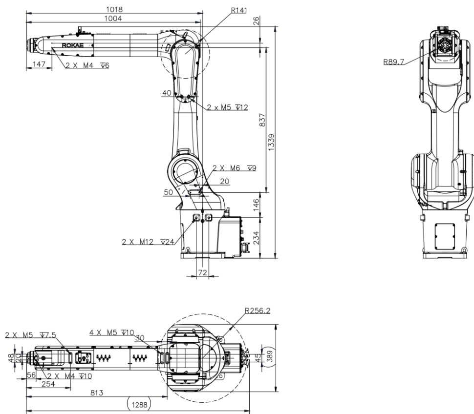
图 17 NB12-10/1.6 外形尺寸及机械接口图
