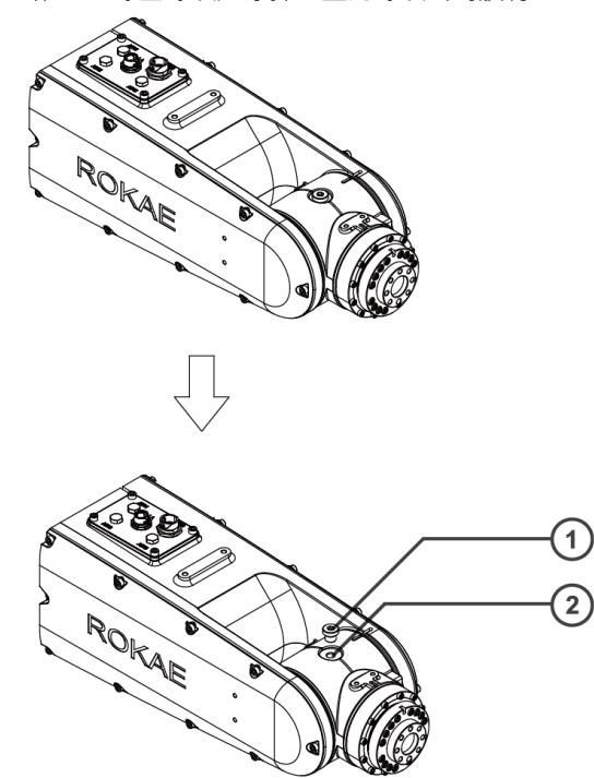
图 47 标准手腕润滑脂加注
