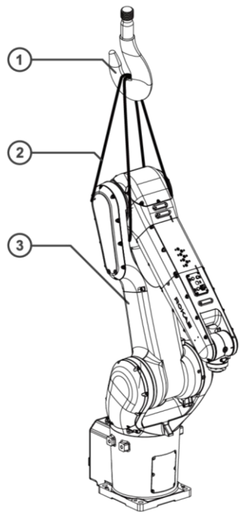
图 25 机器人吊装搬运
