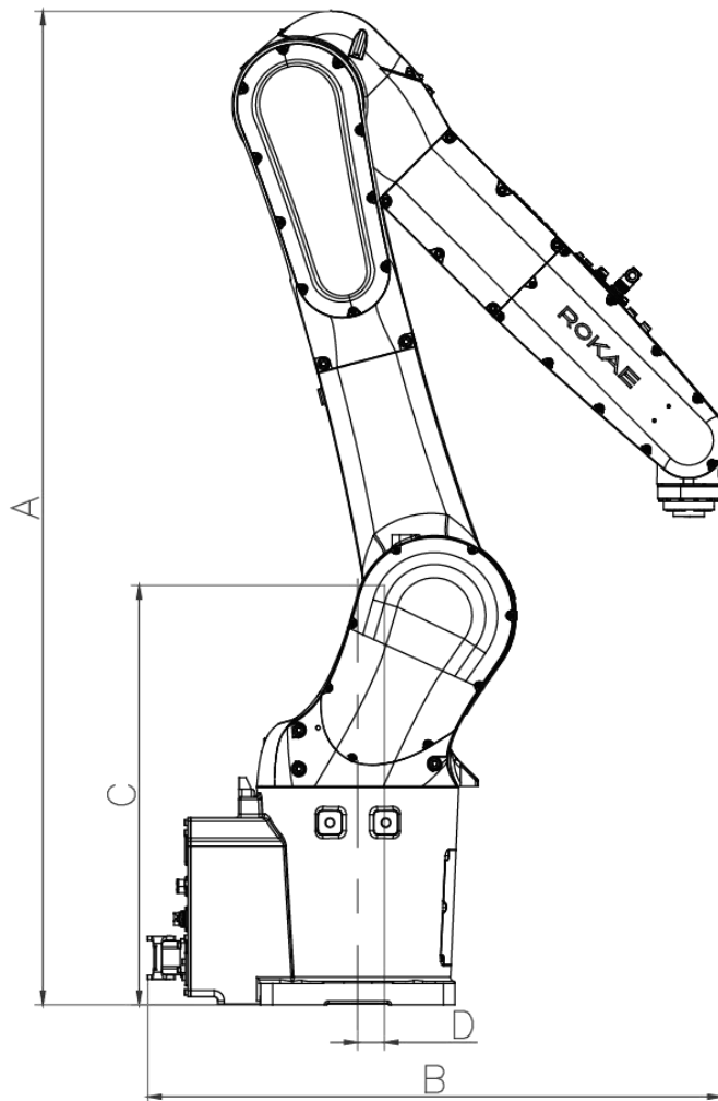
图 24 NB12 系列机器人搬运及重心参考尺寸
