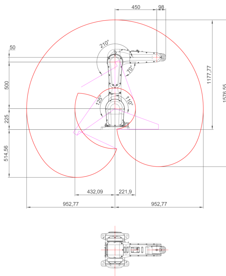
图 13 NB12-16/0.95-3 和 NB12-16/0.95-4 工作空间图
