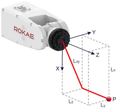
图 7 负载重心
