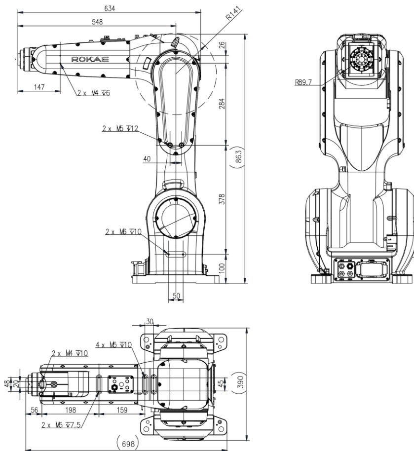
图 18 NB12-16/0.95-3 和 NB12-16/0.95-4 外形尺寸及机械接口图
