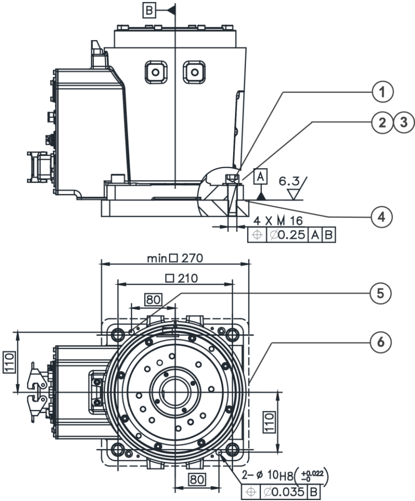
图 27 NB12-12/1.4、NB12-16/1.1、NB12-16/1.0 和 NB12-10/1.6 的支架固定方式
